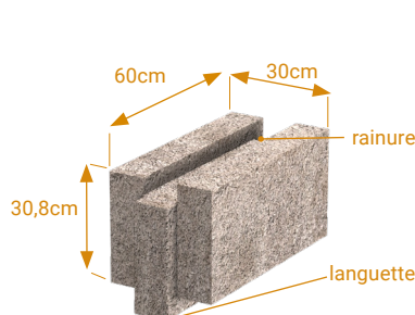
Bloc standard poids : 21 kg
