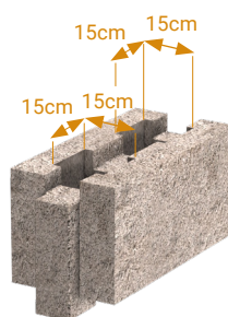
Bloc double poteau poids : 15 kg
