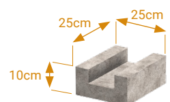
Semelle départ poids : 7,8 kg
