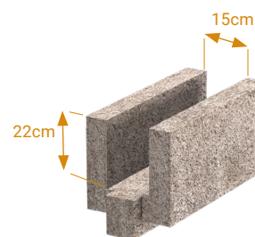
Bloc U chaînage poids : 14 kg
