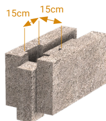
Bloc poteau poids : 16 kg
